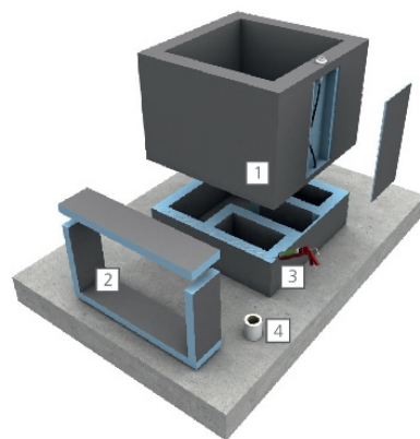
C Réalisation du système : pédiluve
