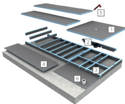
B Réalisation du système : socle
